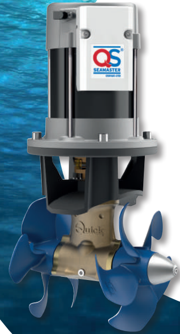
Mod. QSB 160-250
