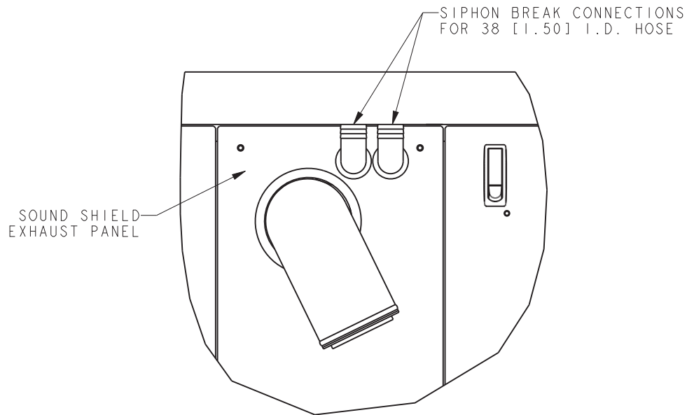
OPTIONAL SIPHON BREAK KIT SCALE 0.250
