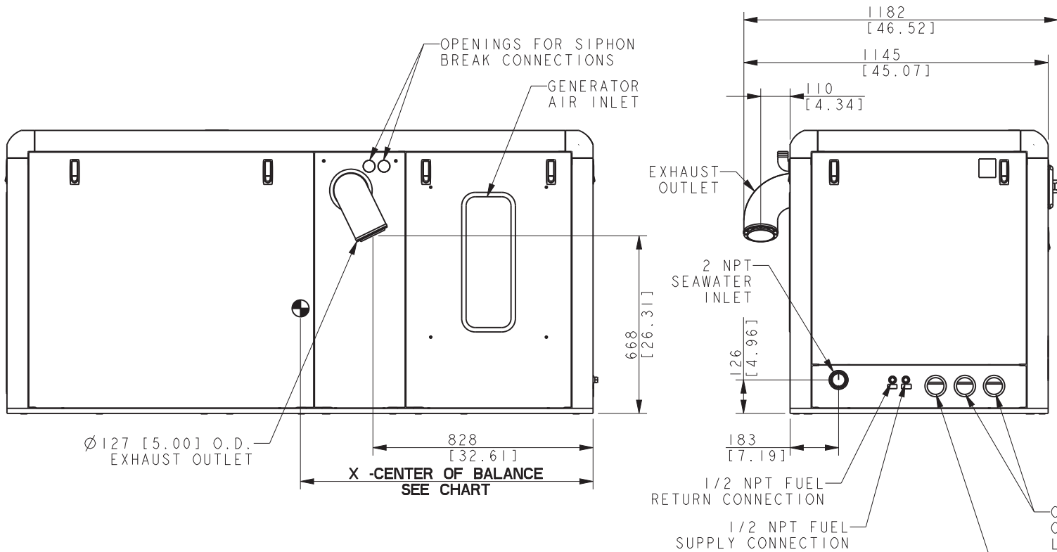
OPTIONAL SIPHON BREAK KIT SCALE 0.250
